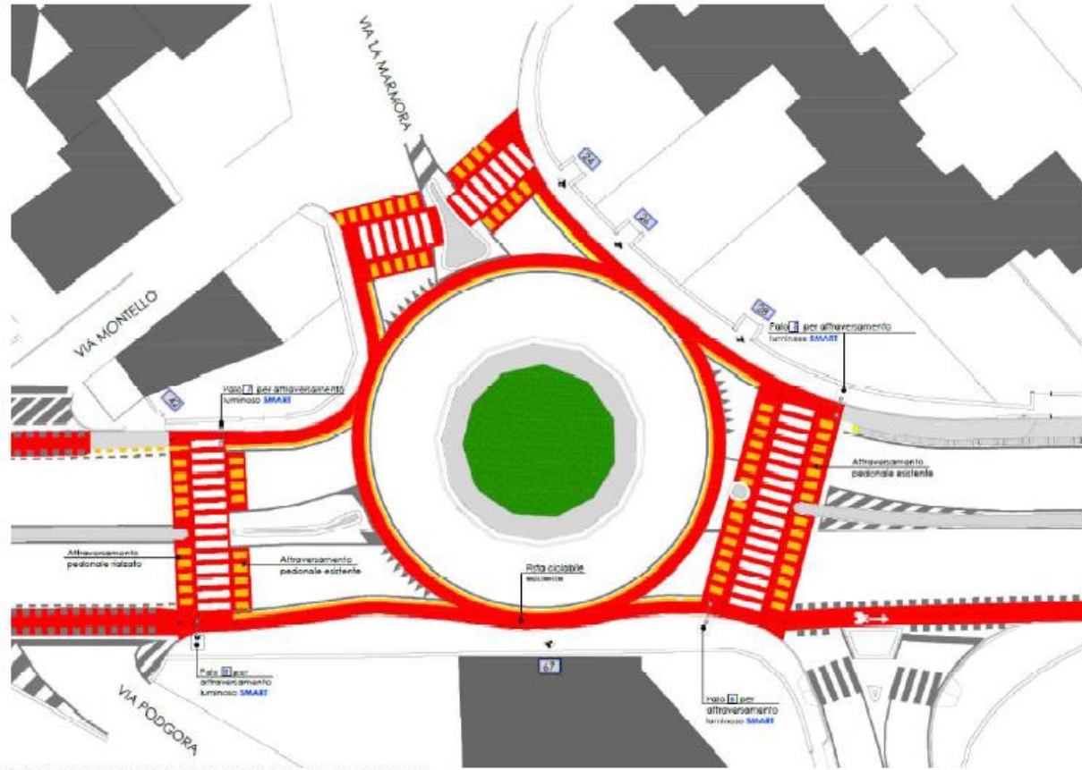
STRALCIO ROTATORIA CORSO ARGENTINA - VIA LA MARMORA
