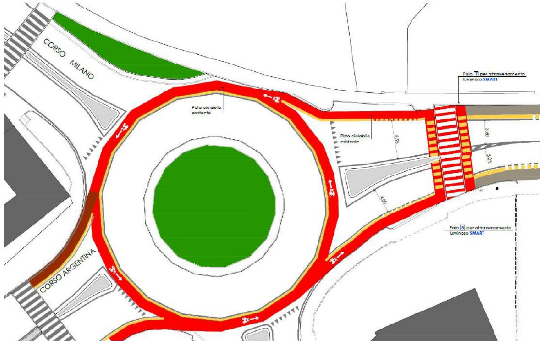
STRALCIO ROTATORIA CORSO MILANO-CORSO ARGENTINA-VIA S.GIOVANNI
