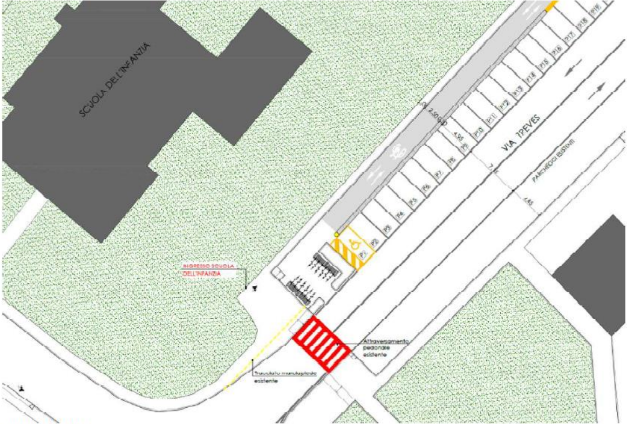
STRALCIO VIA TREVES
