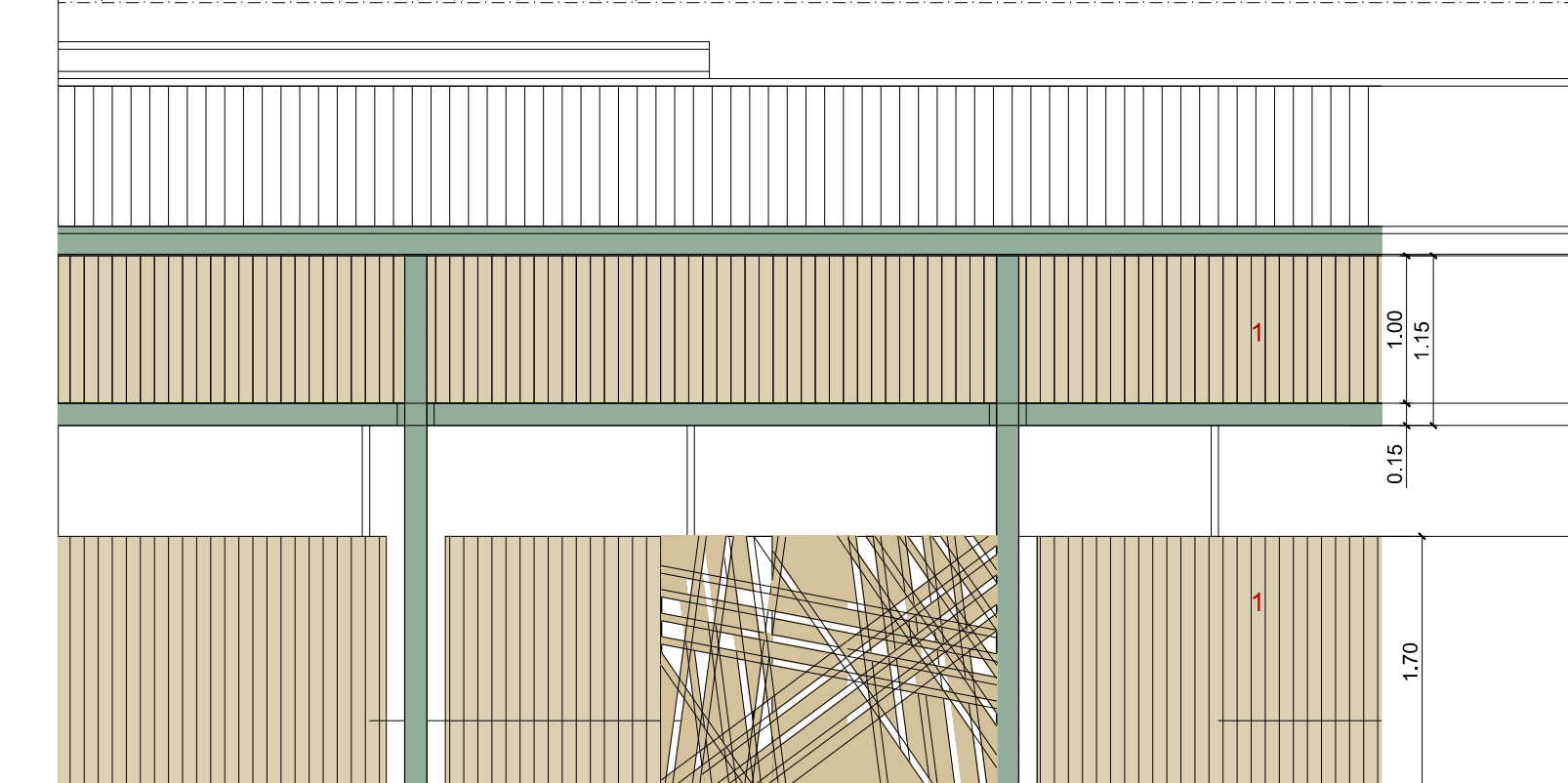
PROSPETTO. DETTAGLIO IN SCALA 1:50 1 PANNELLI CON FUNZIONE FONOASSORBENTE IN MATERIALE CEMENTIZIO
